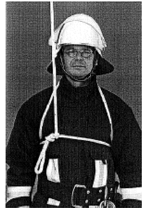
Gesamtansicht Brustbund
